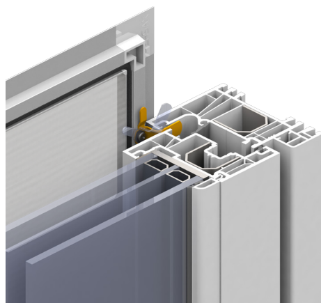
Detalle de la unión al conjunto de la carpintería
