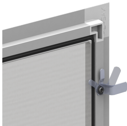
Sistema de CLIPADO directamente a la carpintería
